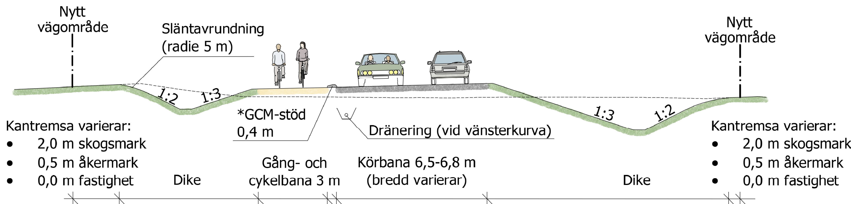
TYPSEKTION, GÅNG- OCH CYKELVÄG SEPARERAS FRÅN KÖRBANA MED GCM-STÖD SKALA 1:100
