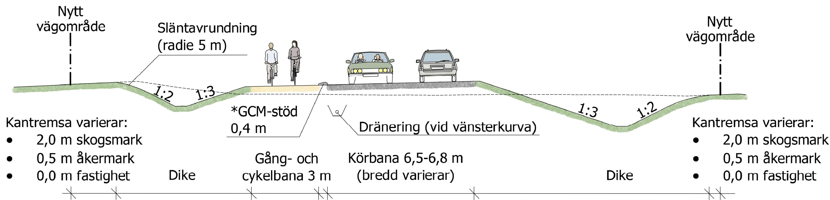
TYPSEKTION, GÅNG- OCH CYKELVÄG SEPARERAS FRÅN KÖRBANA MED GCM-STÖD SKALA 1:100
